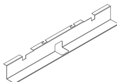
SG16 1160 / 107 / 120 3 kg
