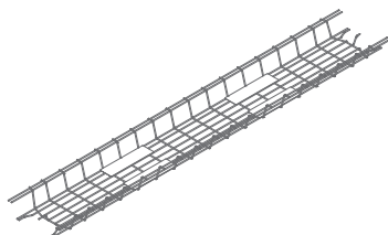
SOD20 2000 / 290 / 77 4 kg
