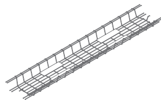
SOD18 1800 / 290 / 77 3,5 kg
