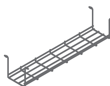
S69 580 / 162 / 123 1 kg
