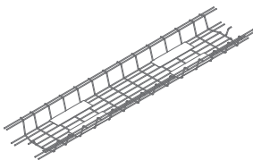
SOD16 1600 / 290 / 77 3 kg
